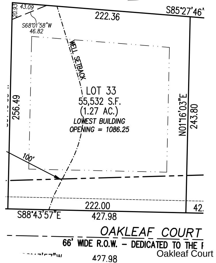
Plat N.T.S
