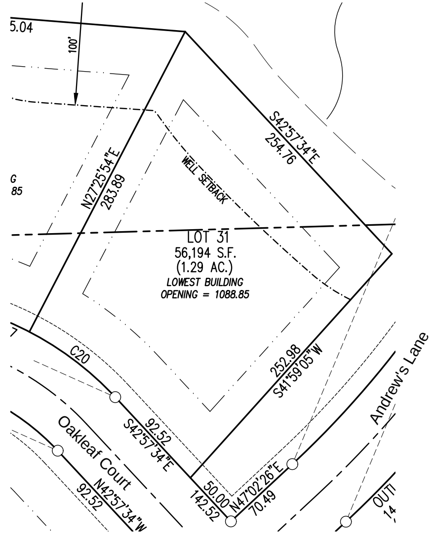
Plat N.T.S.
