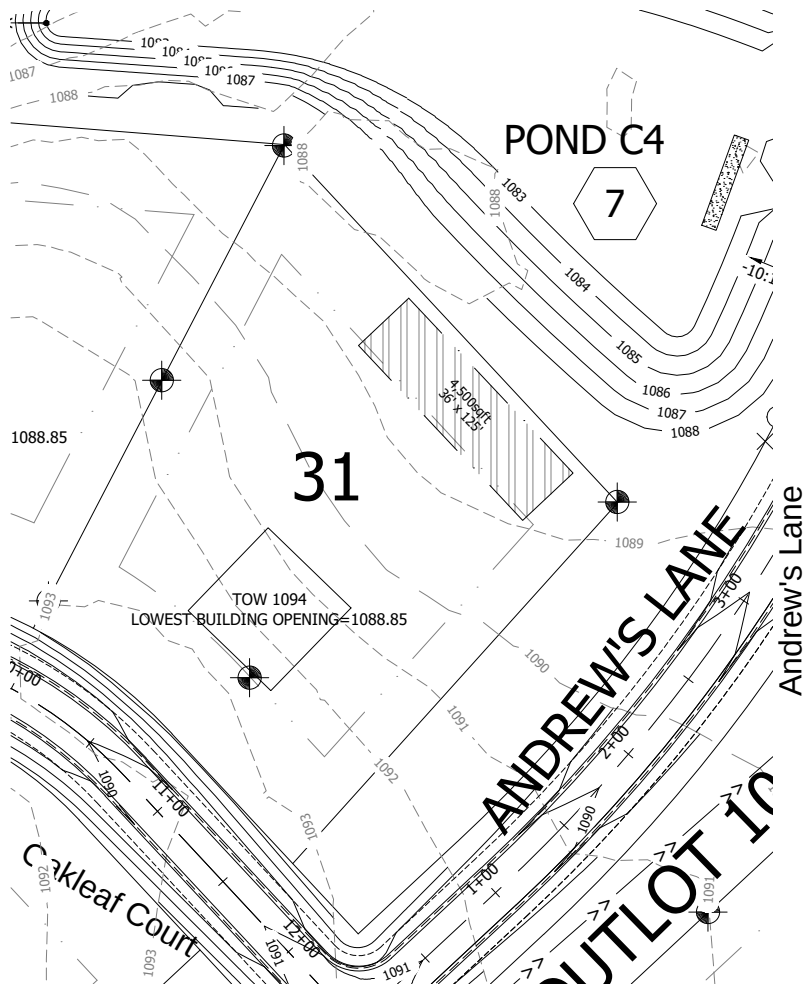
Grading Plan N.T.S.
