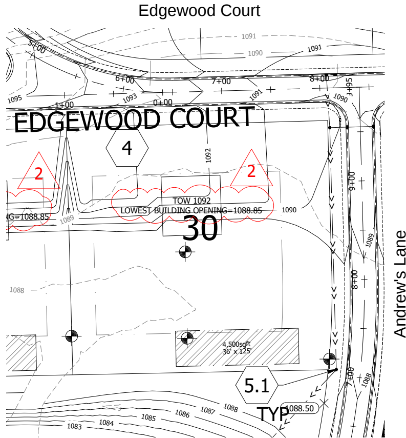
Grading Plan N.T.S
