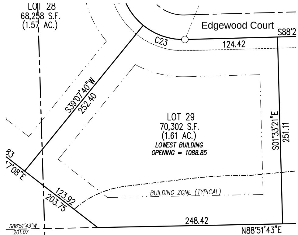
Plat N.T.S
