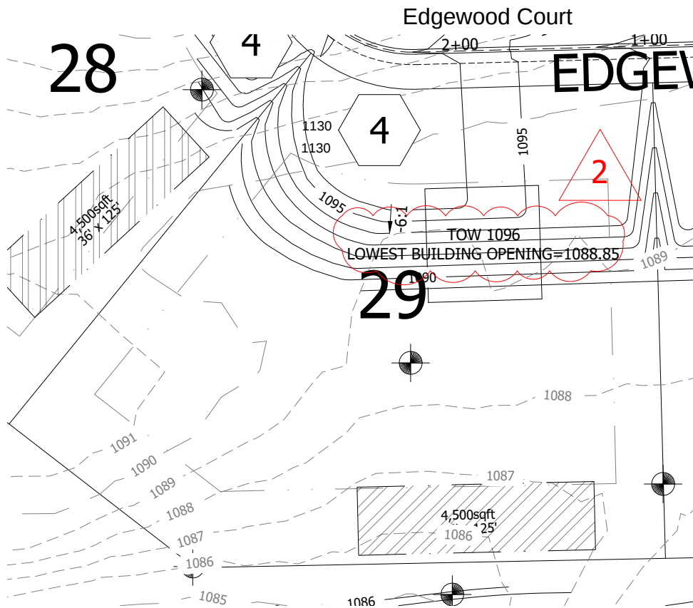
Grading Plan N.T.S
