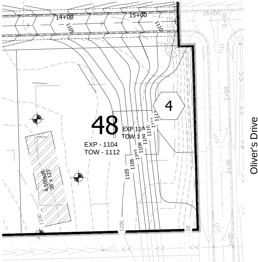
Grading Plan N.T.S
