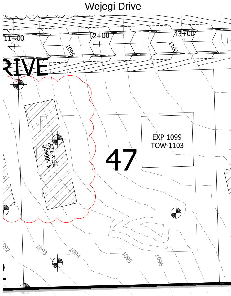
Grading Plan N.T.S.
