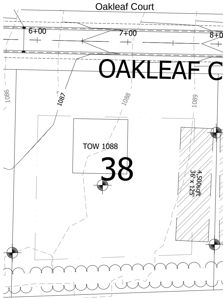
Grading Plan N.T.S
