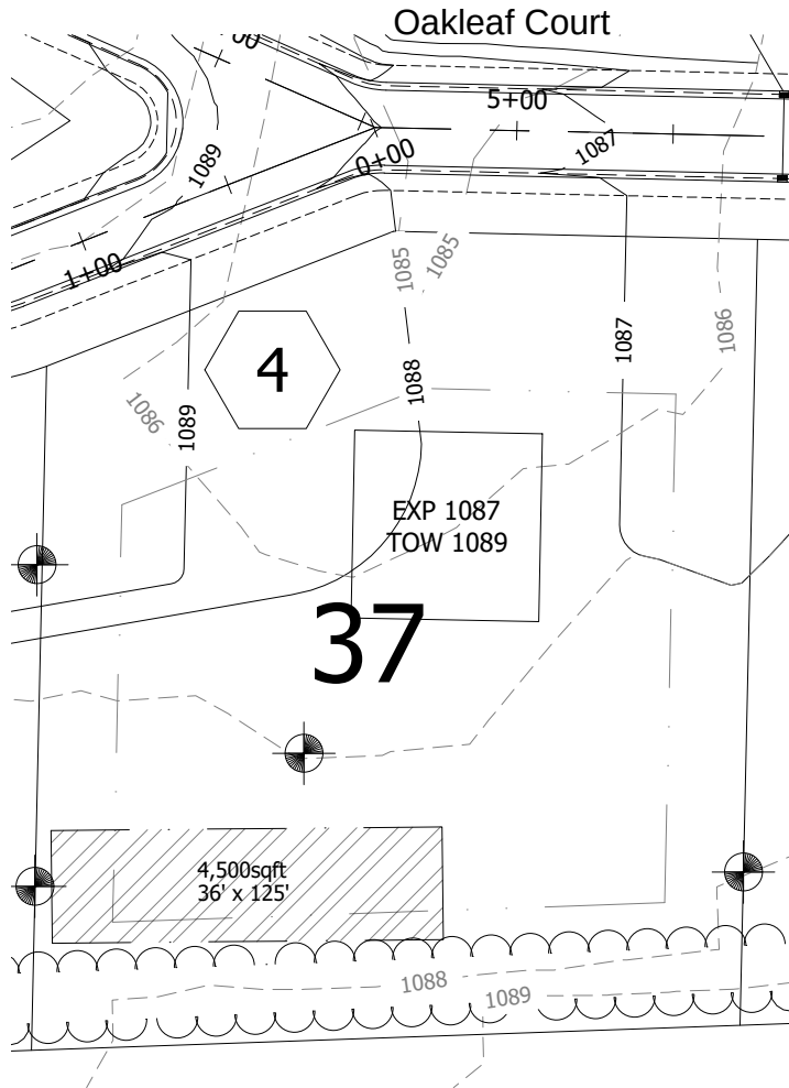
Grading Plan N.T.S
