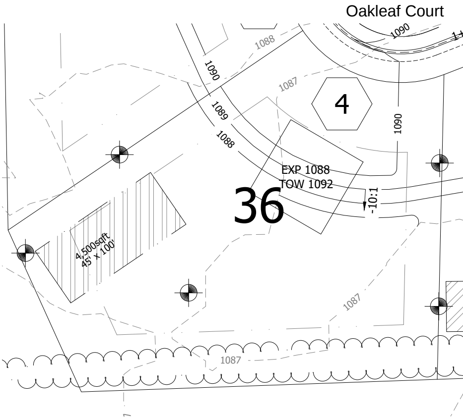
Grading Plan N.T.S
