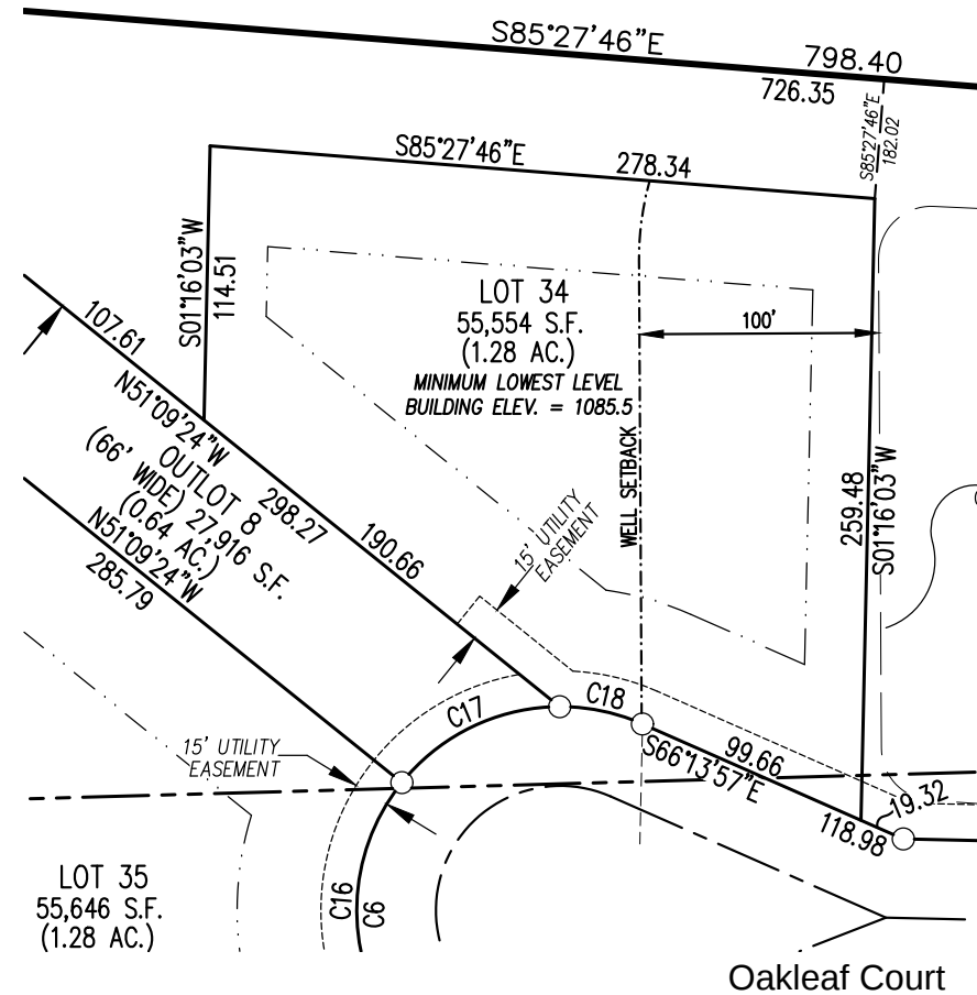
Plat N.T.S
