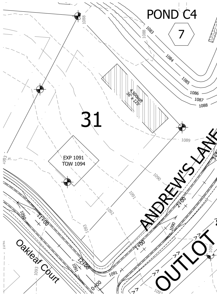
Grading Plan N.T.S
