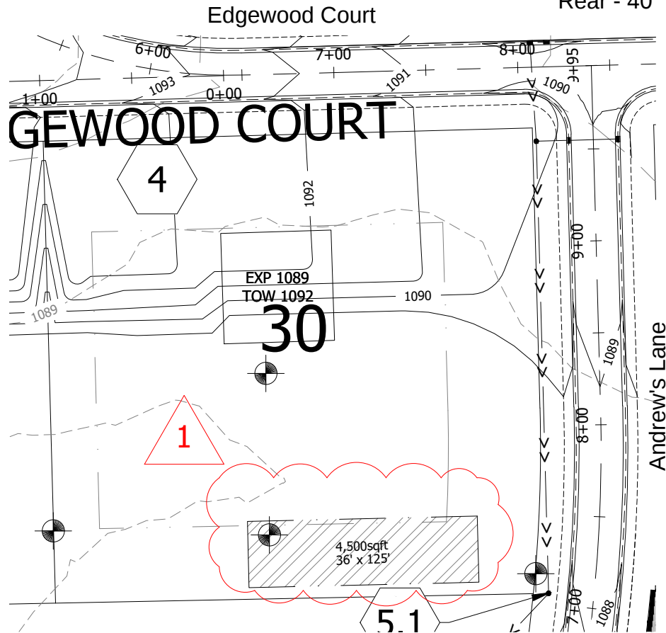
Grading Plan N.T.S
