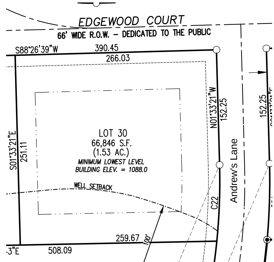
Plat N.T.S
