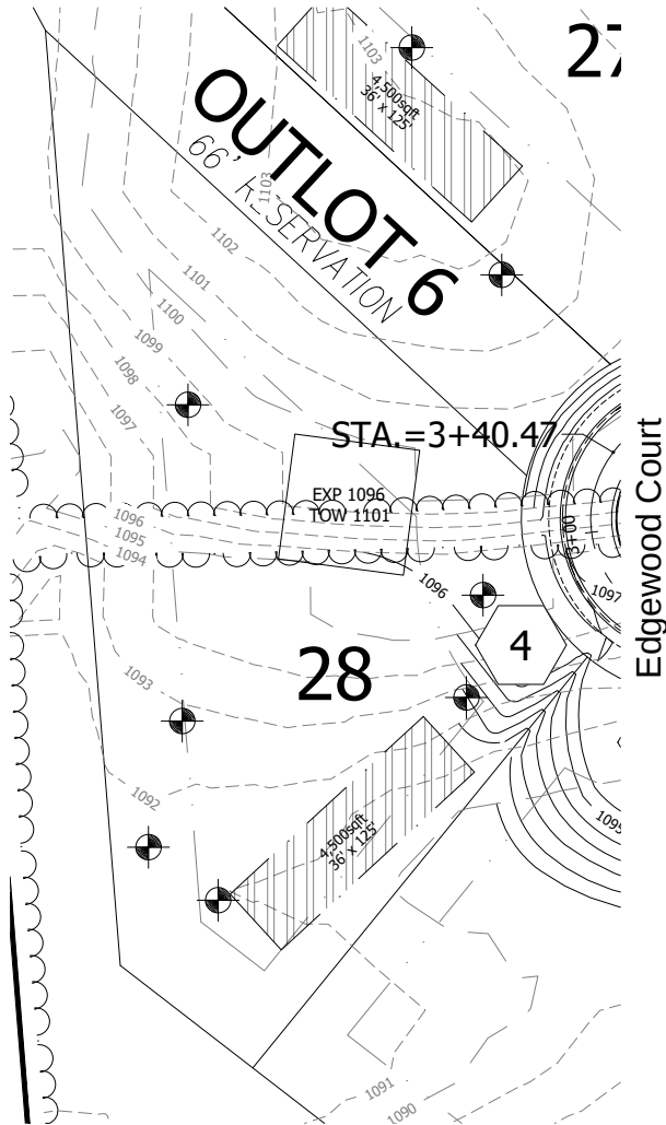
Grading Plan N.T.S
