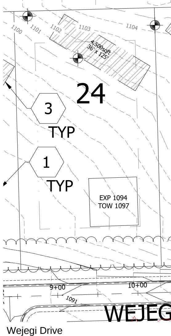
Grading Plan N.T.S
