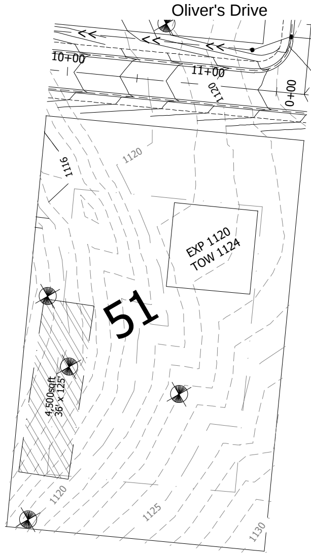
Grading Plan N.T.S.
