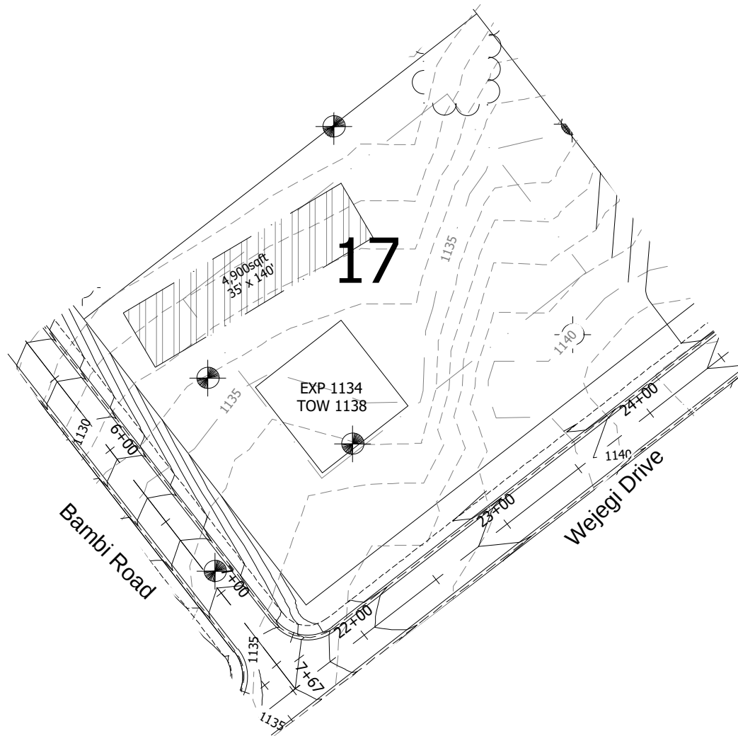
Grading Plan N.T.S
