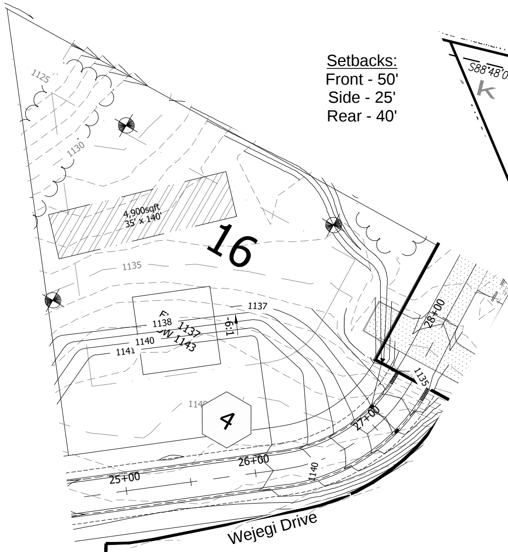
Grading Plan N.T.S
