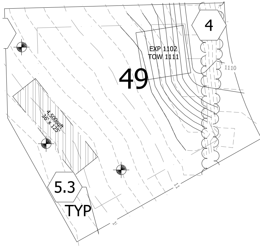
Grading Plan N.T.S
