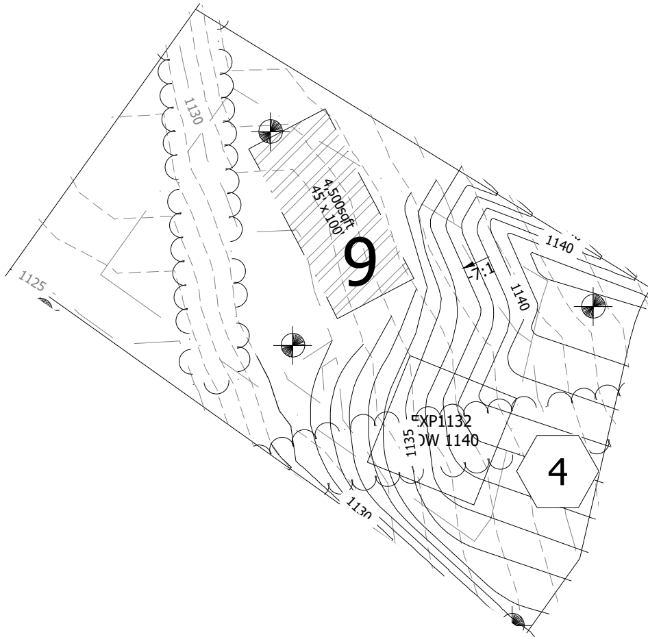
Grading Plan N.T.S
