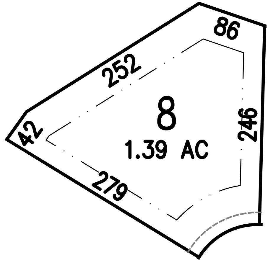
Plat N.T.S
