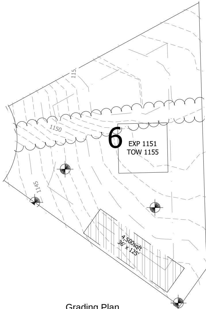
Grading Plan N.T.S
