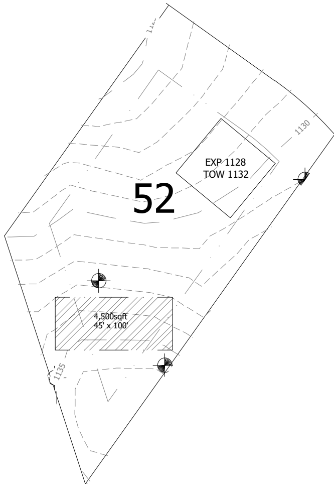
Grading Plan N.T.S
