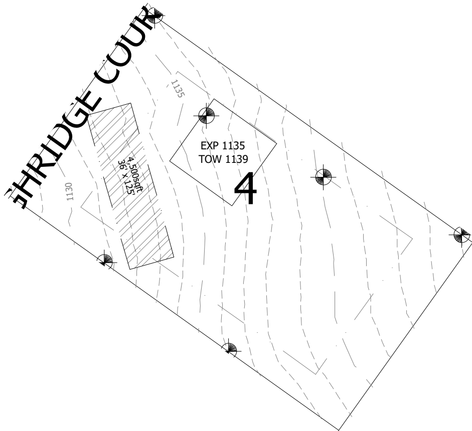
Grading Plan N.T.S
