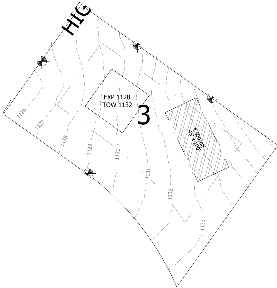
Grading Plan N.T.S
