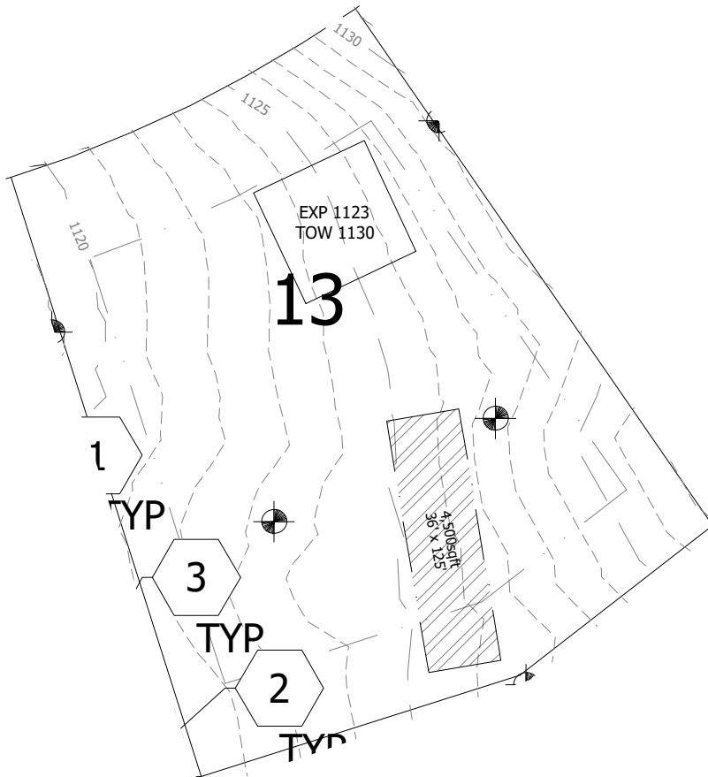
Grading Plan N.T.S
