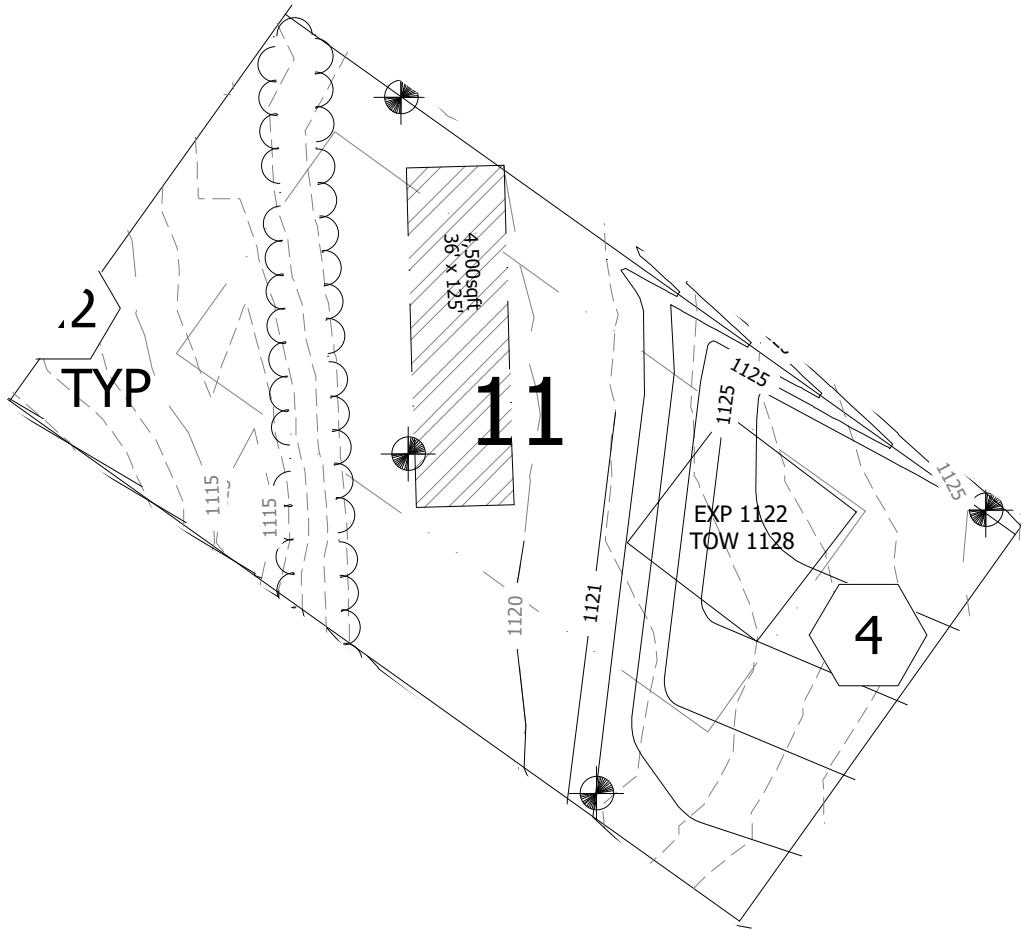
Grading Plan N.T.S
