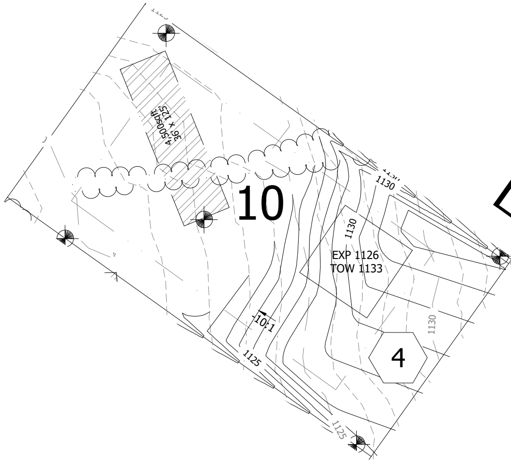
Grading Plan N.T.S
