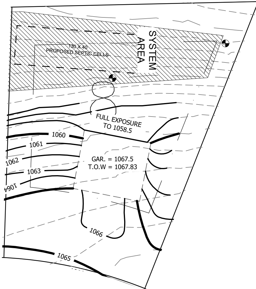
Grading Plan N.T.S
