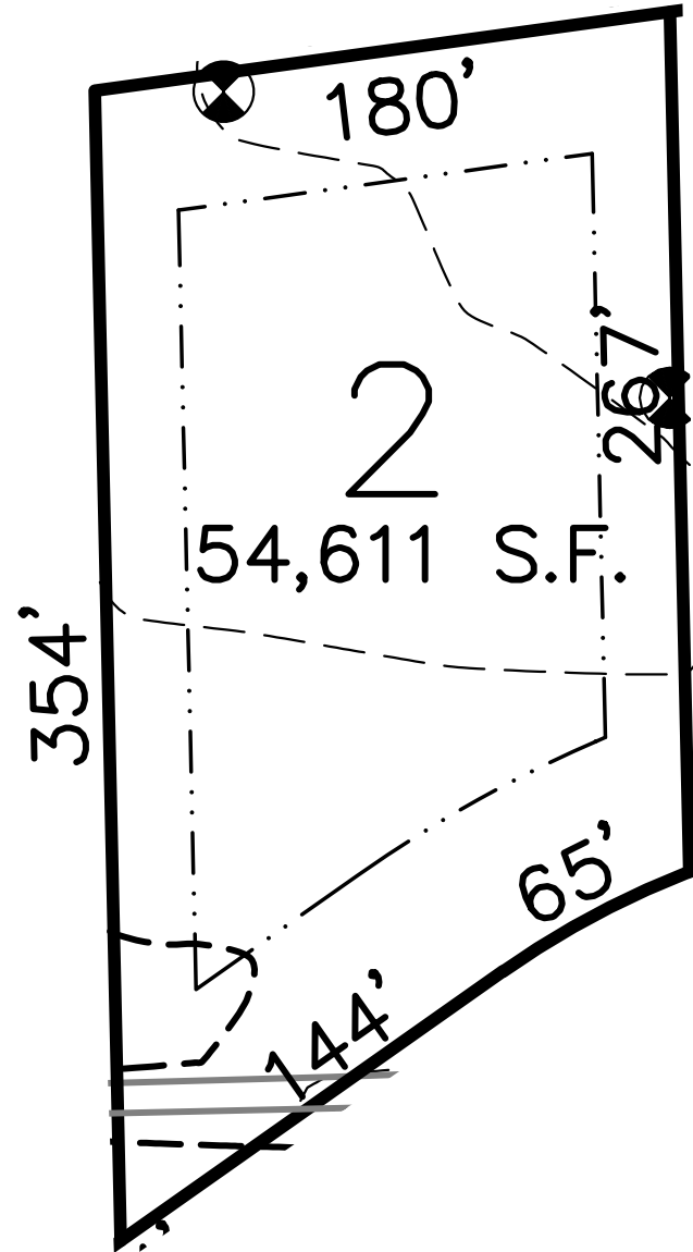
Plat N.T.S
