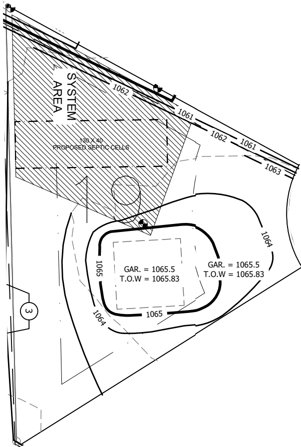
Grading Plan N.T.S
