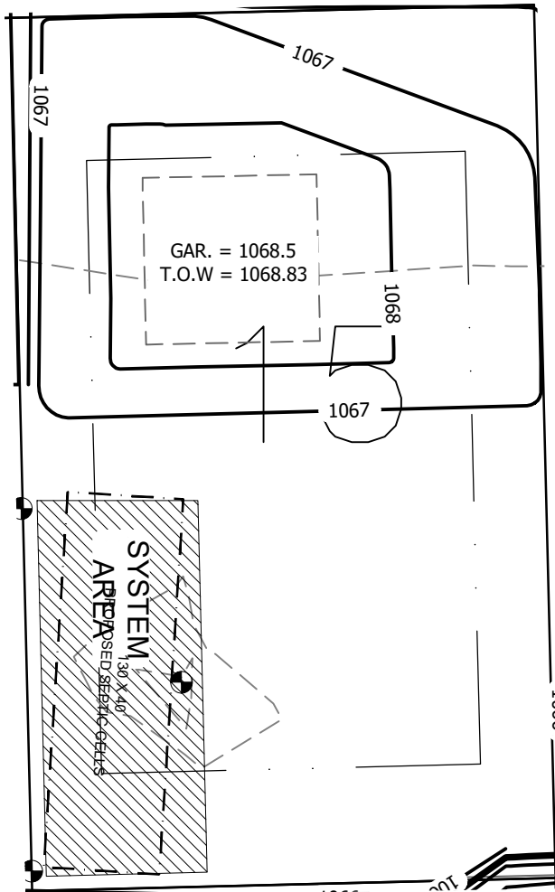
Grading Plan N.T.S
