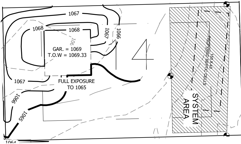
Grading Plan N.T.S
