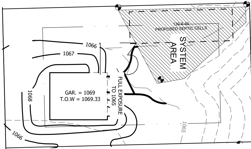
Grading Plan N.T.S
